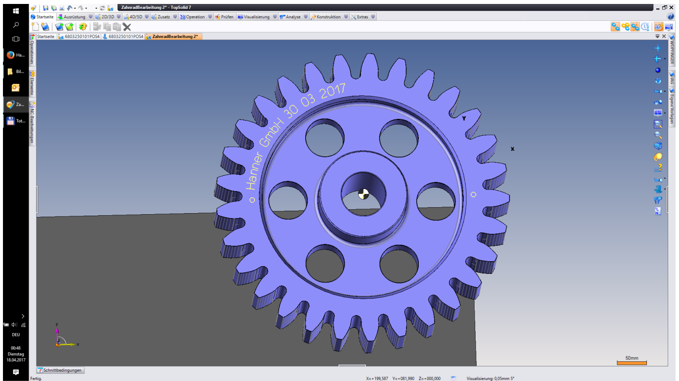
Zahnrad m16/ z29 Durchmesser 500mm
