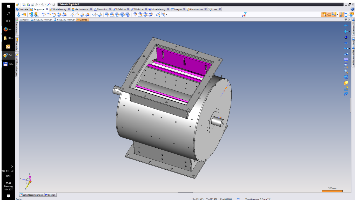
Zellradschleuse Durchmesser 800mm mit Verschleißauskleidung aus
